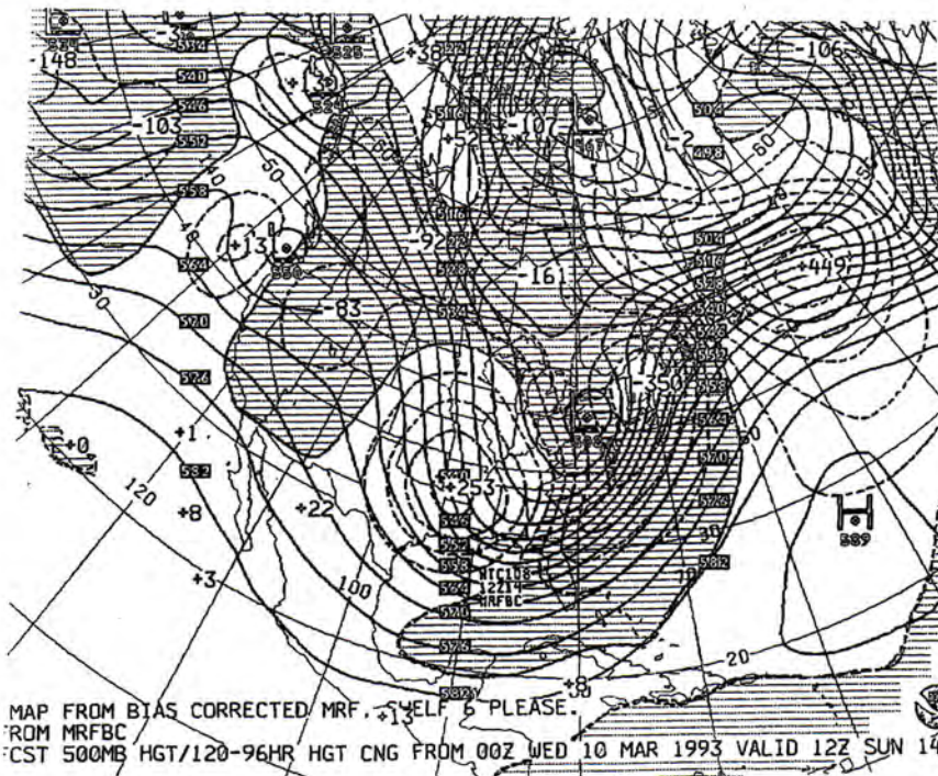
500 mb
